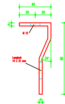
Befestigungswinkel Maßstab 1 : 5
