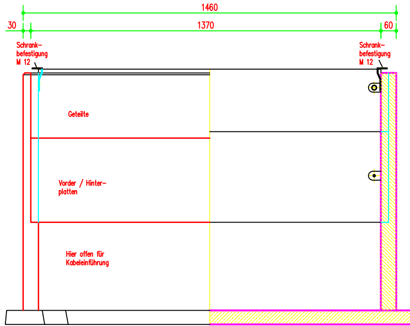
Vorderansicht / Schnitt
